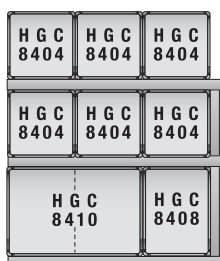
UNIT 26 幅1,990mm/高さ2,180mm
